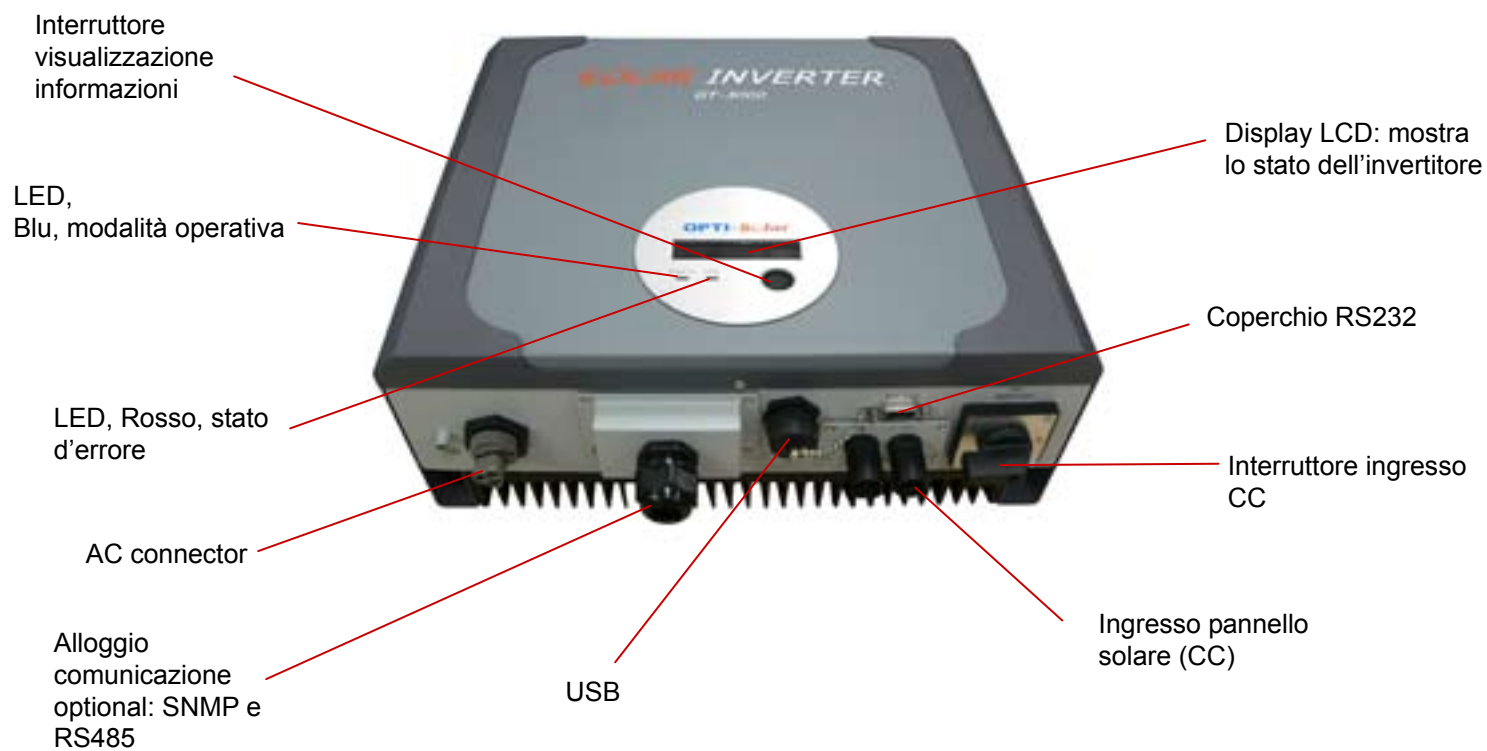
Veduta frontale
